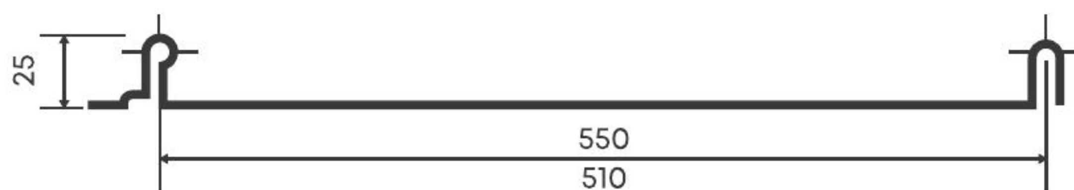
Фальцевая кровля
